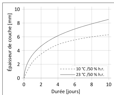
Diagramme 1: Vitesse de durcissement de Sikaflex®-552 AT
