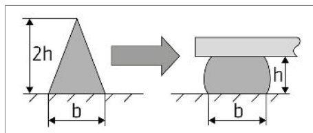
Croquis 1: Application de colle recommandée
