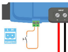
a) Câblage des broches L-H
