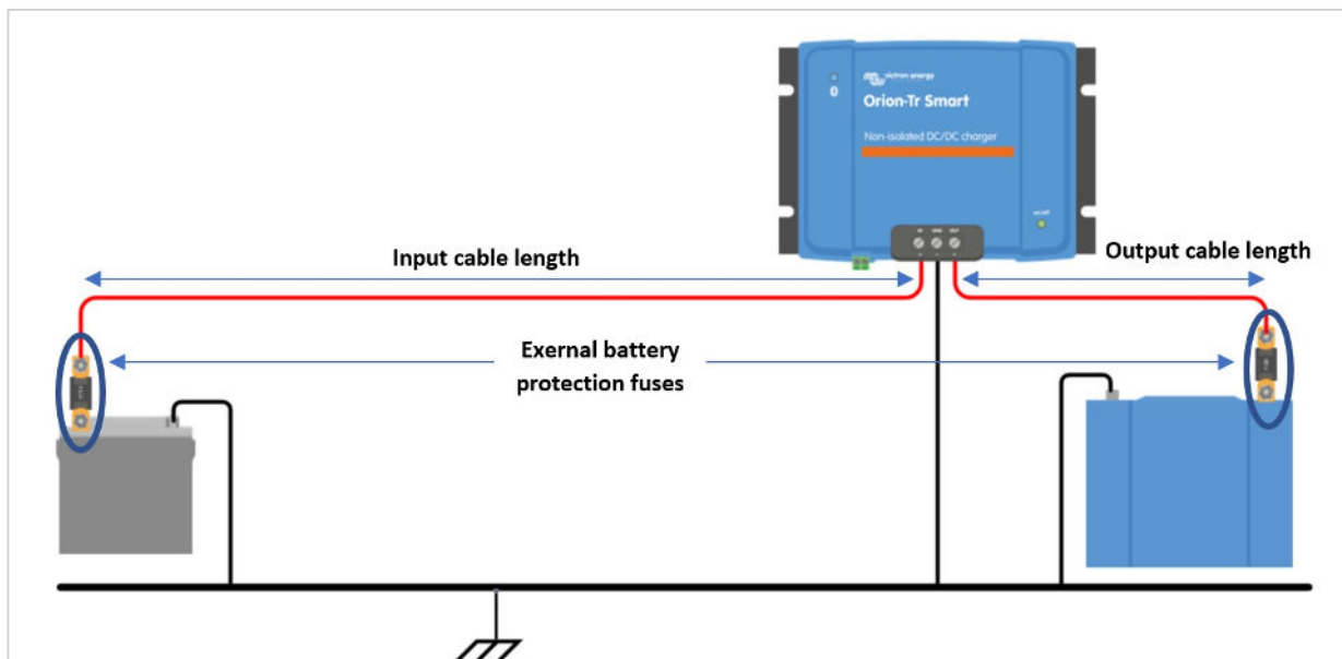
Illustration 6 : Recommandations relatives aux câbles et aux fusibles
