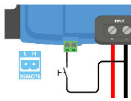
c) Câblage de la broche L
