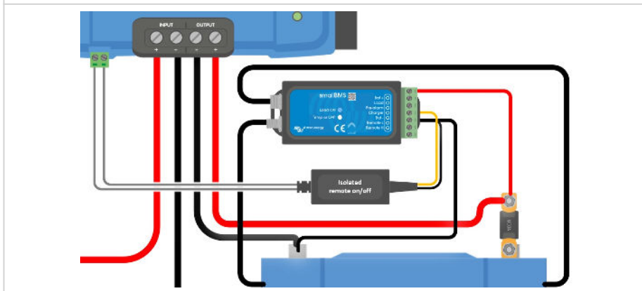
d) Câble isolé d'allumage/arrêt à distance
