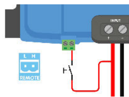
d) Câble isolé d'allumage/arrêt à distance
