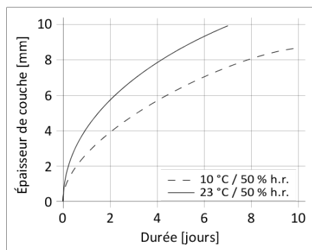
Diagramme 1: Vitesse de durcissement
