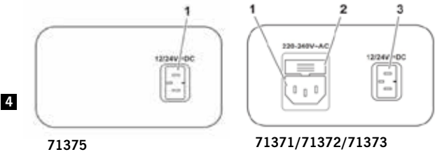
Anschlussbuchsen, Abb. 4
