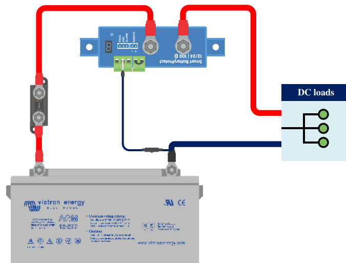
Smart BatteryProtect dans un système simple avec un cavalier entre les entrées L et H (réglage d'usine)
