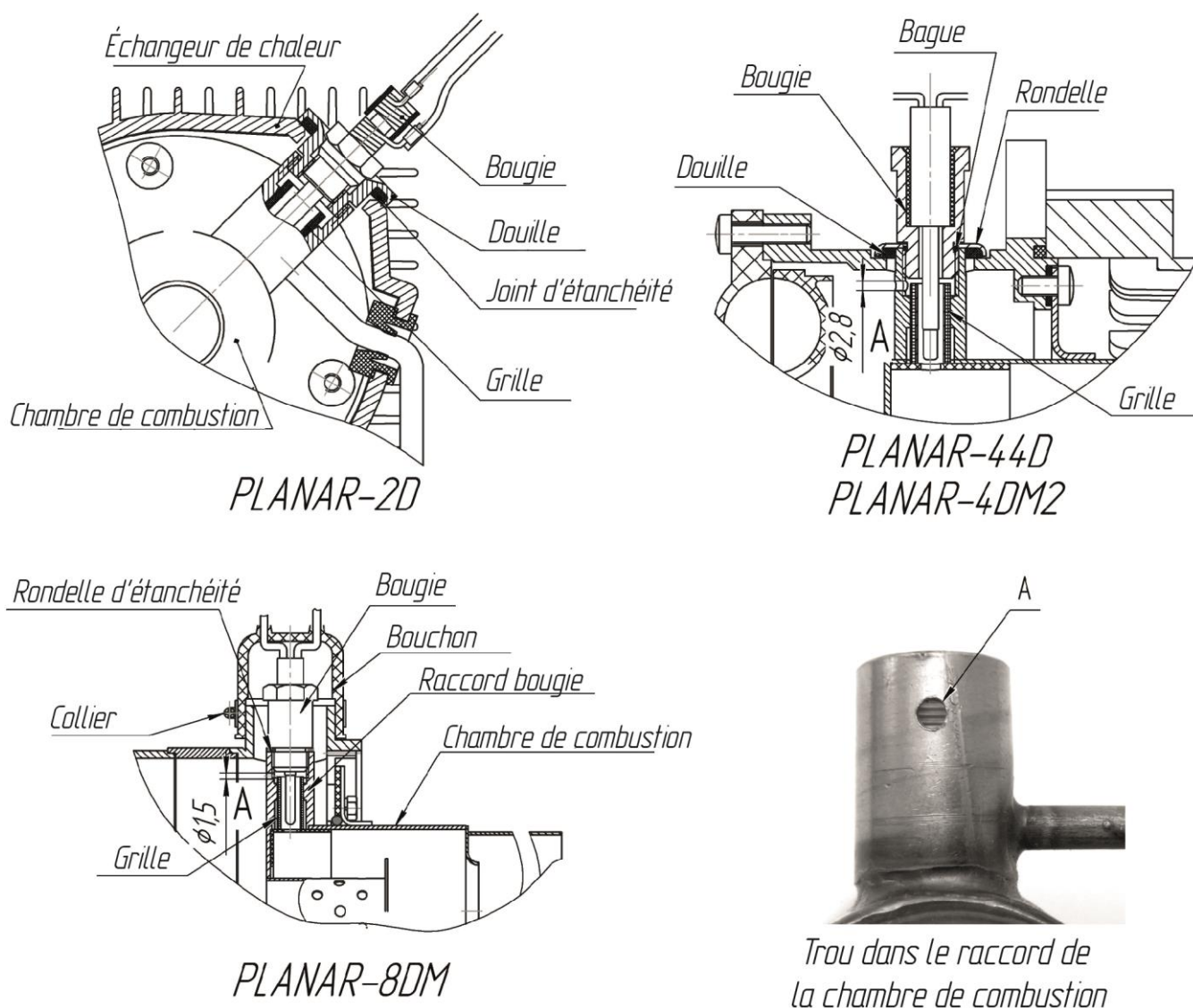
Fig.5 – Schéma d'installation de la bougie et de la grille dans le raccord de la chambre de combustion
