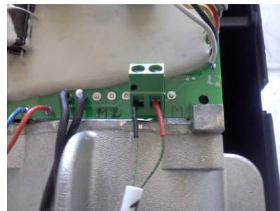
Fig. 9a – Connexion
