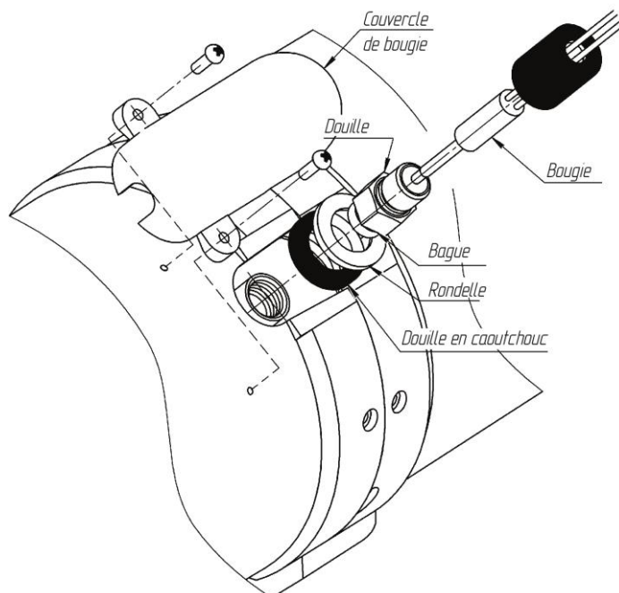
Fig.4 - Bougie avec un kit de montage
