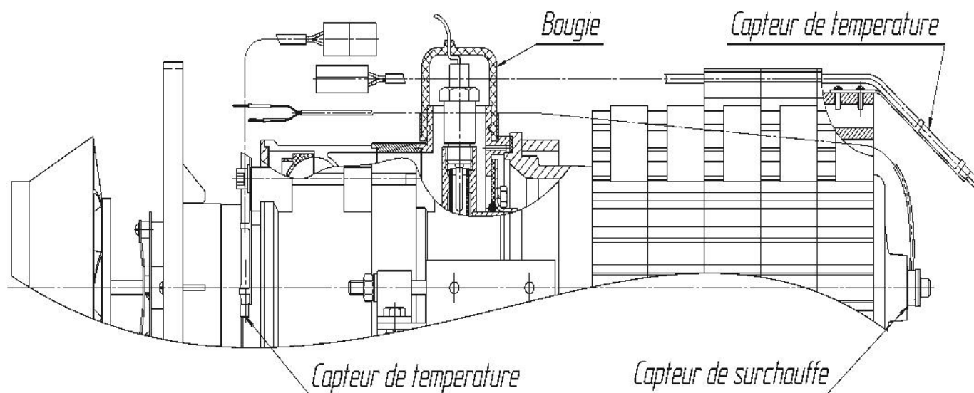
Fig.10 - Capteurs
