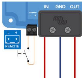
a) Câblage des broches L-H
