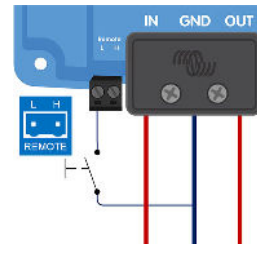
c) Câblage de la broche L
