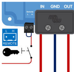
Diagramme de connexion pour ignorer la détection de moteur à l'arrêt
