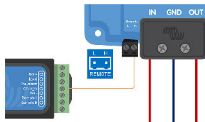
d) Contrôle du BMS via la broche H
