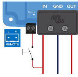
d) Contrôle du BMS via la broche H
