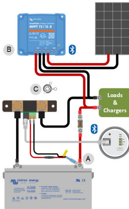
Exemple d'un système contenant un contrôleur de batterie avec une sonde de température et un chargeur solaire, les deux utilisant le réseau VE.Smart.
