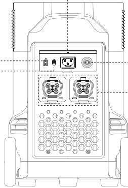
Port d'entrée de charge CA X-Stream
