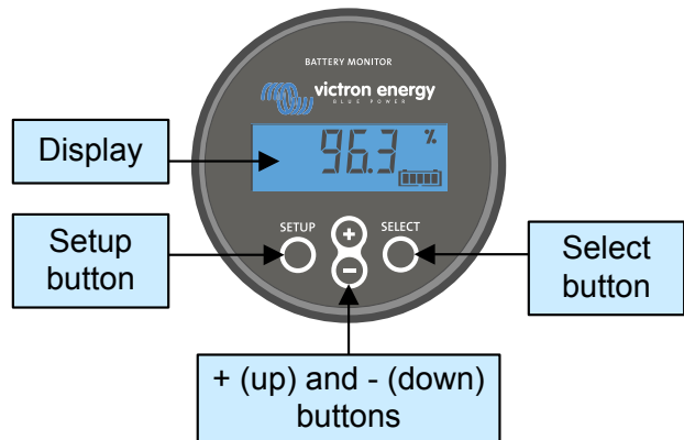
Écran et boutons de l'unité BMV.
